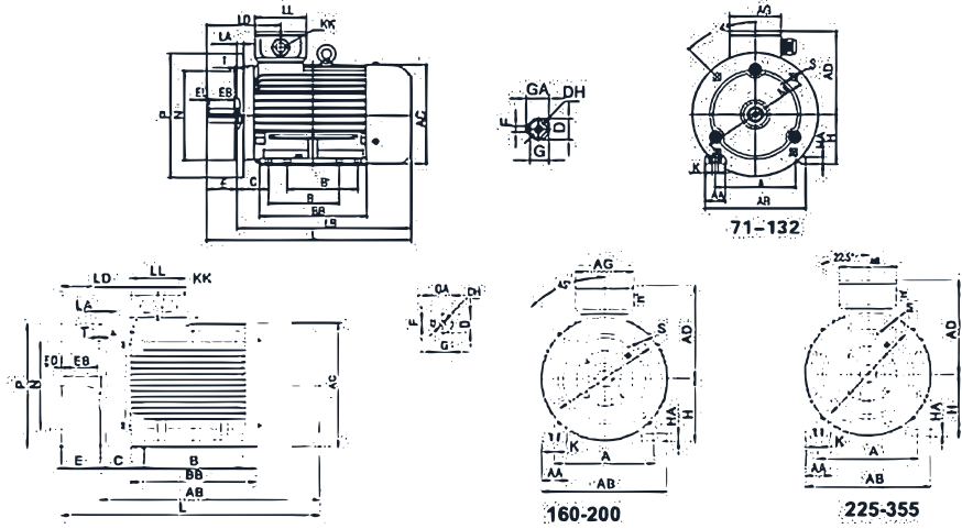
IM B35 — Ayaklı gövde + flanş
