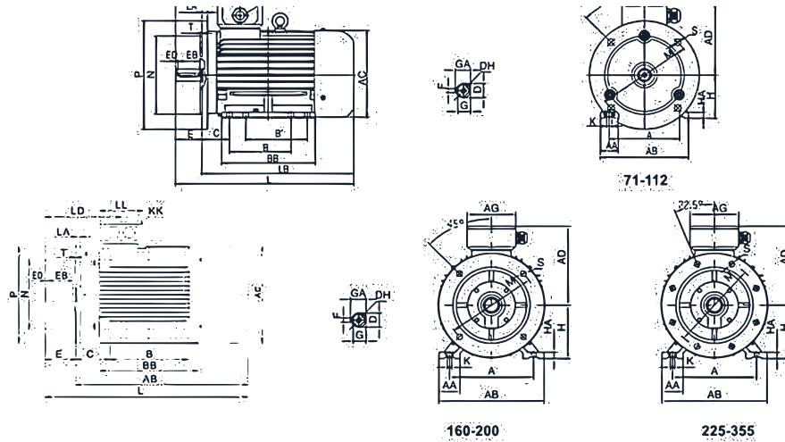
IM B35 — Ayaklı gövde + flanş
